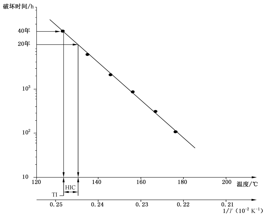
图 A.2 计算老化寿命、温度指数与半差的耐热曲线
