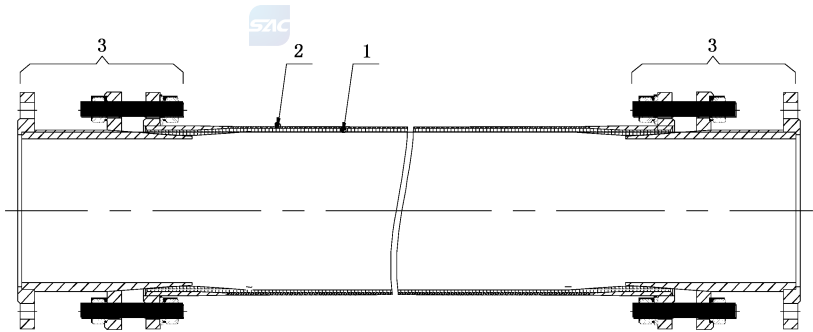
图 3 卡箍接头管件典型结构示意图
