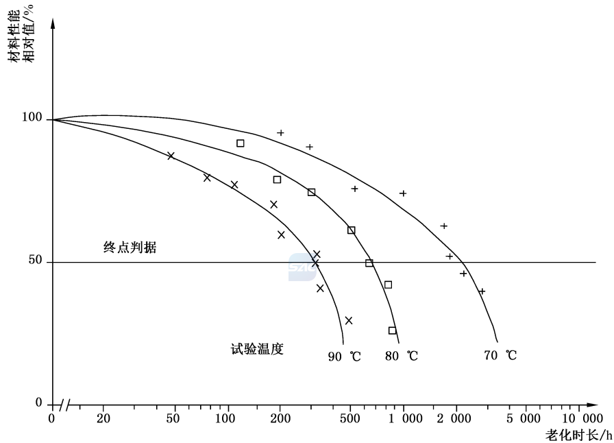
图 A.1 不同温度热水老化条件下的拉伸强度变化图
