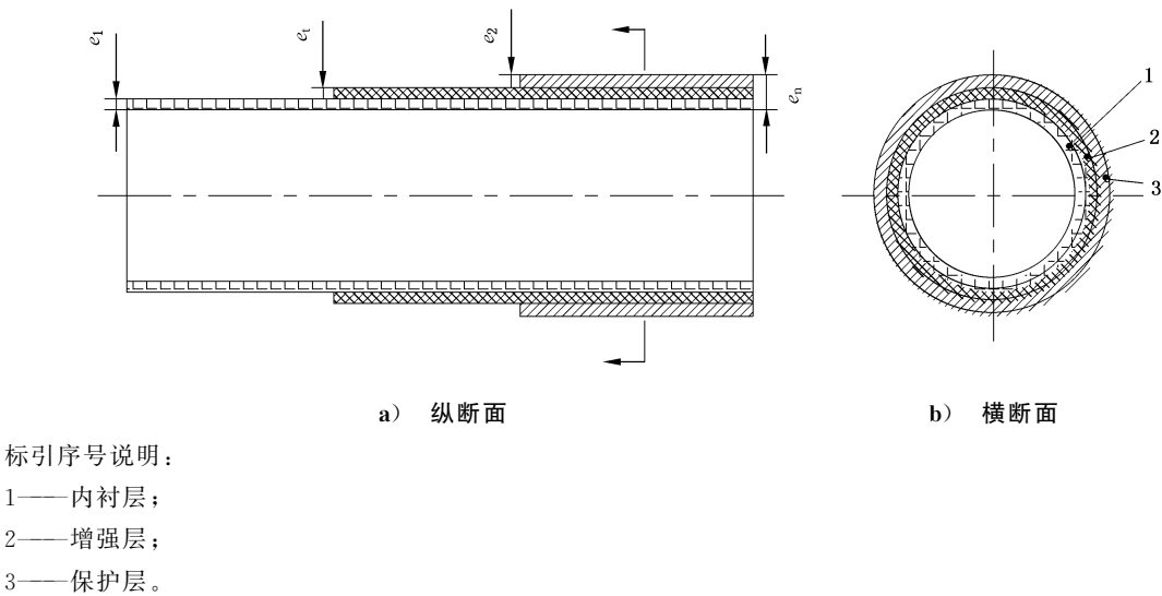
图 2 软管结构示意图
