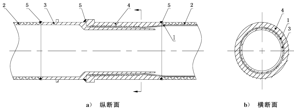
图5 注胶接头管件典型结构示意图
